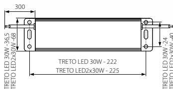
● TRETO LED2x30W
